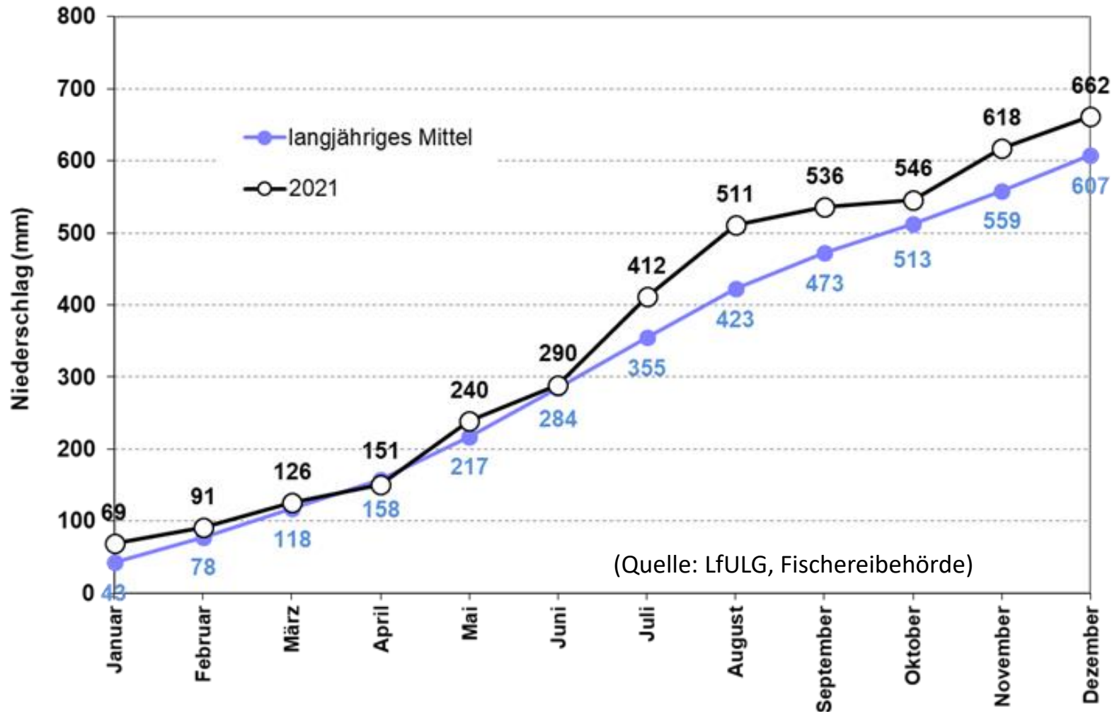
Niederschlagssummenreihe 2021 im Vergleich zum langjährigen Mittel der Niederschlagssummenreihe für Königswartha
